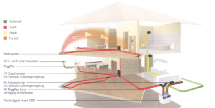
Kontrollierte Wohnraumlüftung
